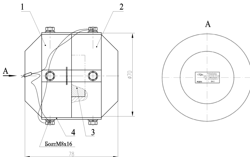
Рис. 5. Кассета СН-1 (СН-2) с установленной транспортной заглушкой.
